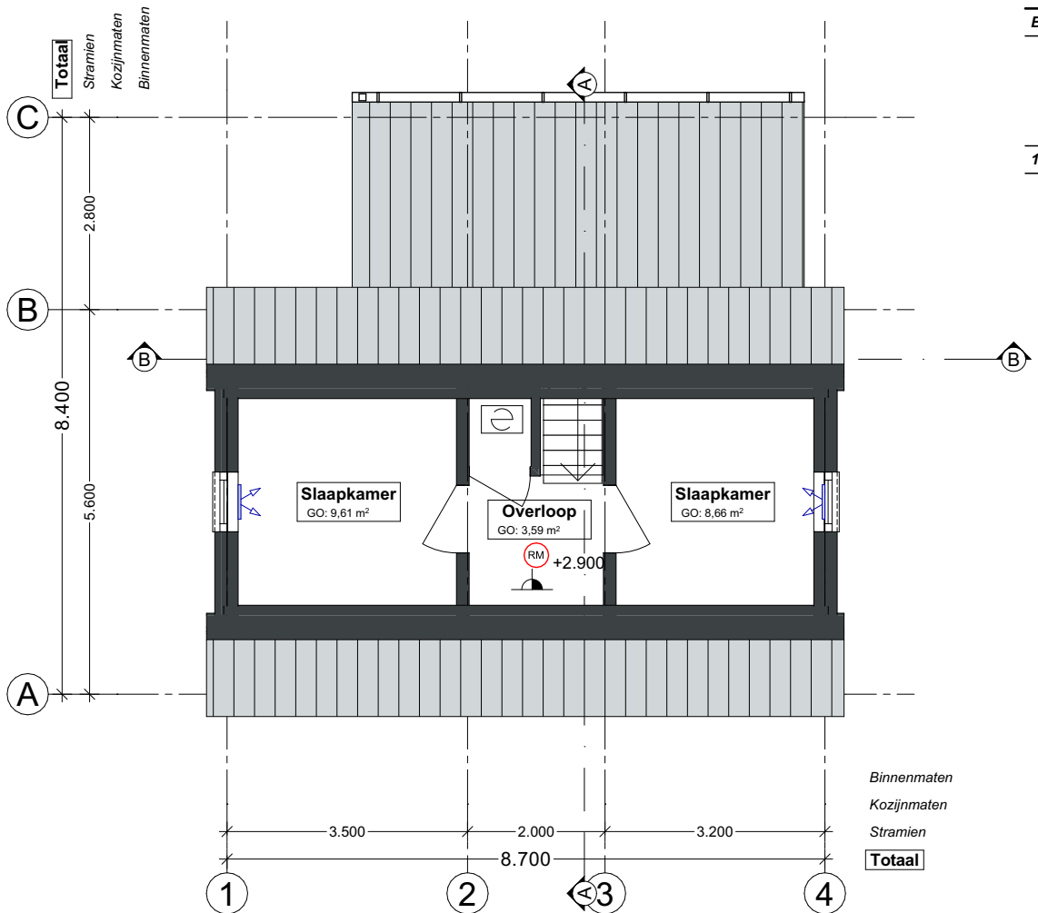
1e verdieping
