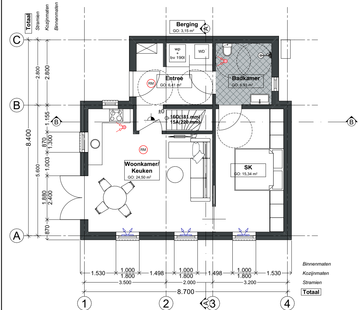
Begane grond
