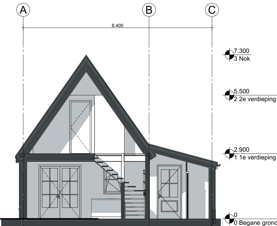
Doorsnede A-A
