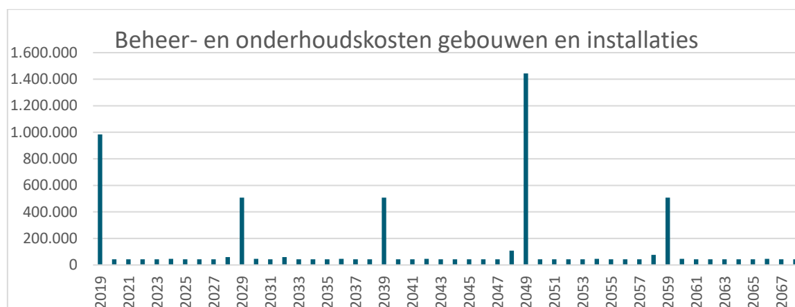
Afbeelding 6.1 Investeringskosten beheergebied gebouw en installaties per jaar
